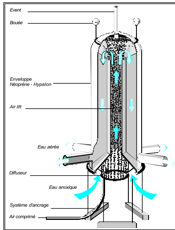
Schéma de principe du LIMNO
